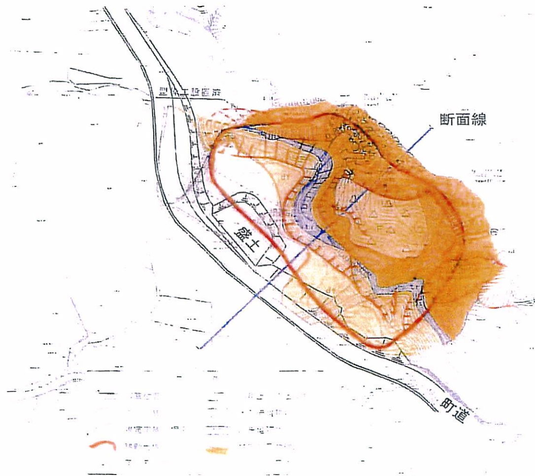
図一12 横壁小倉地区平面図
