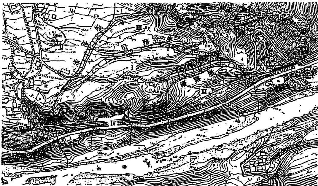
図1-23 林付近の地すべり 中之条土木事務所(1991)による
