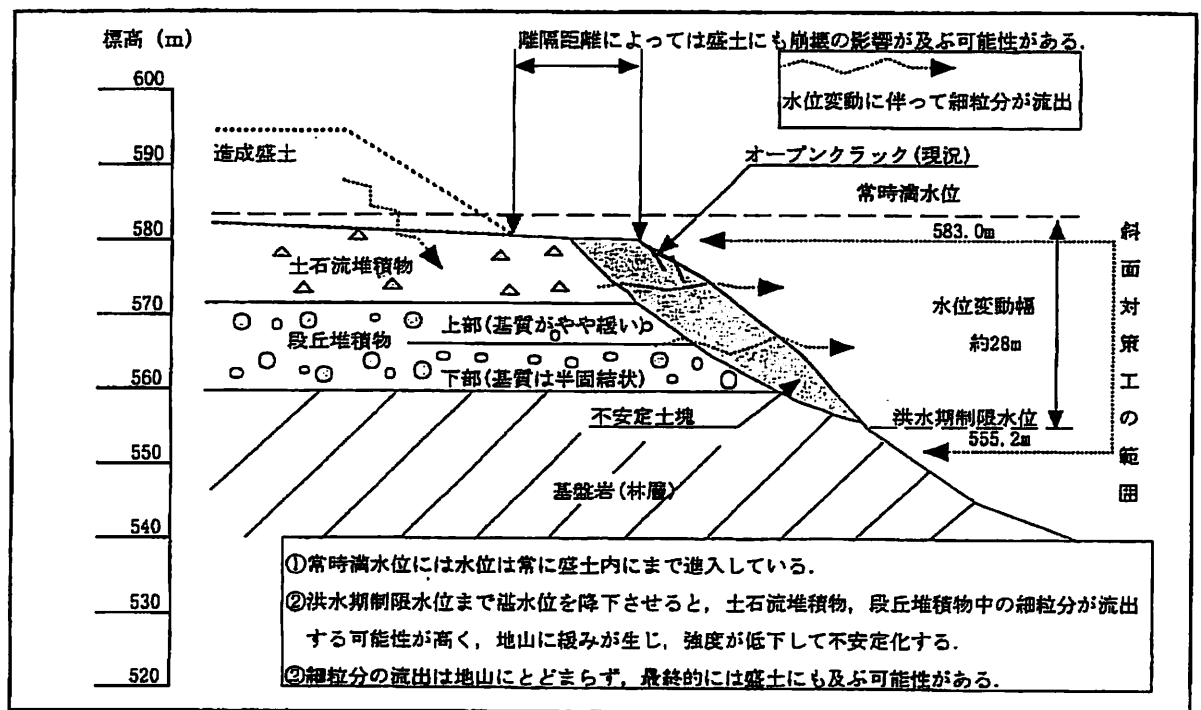
図 V. 1. 1. 4 西久保地区河岸斜面の構造と土木地質的問題点
